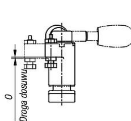
Mocowanie powierzchni poddanych obróbce
