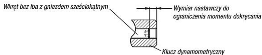
Łapy szybkomocujące K0910.3240...
